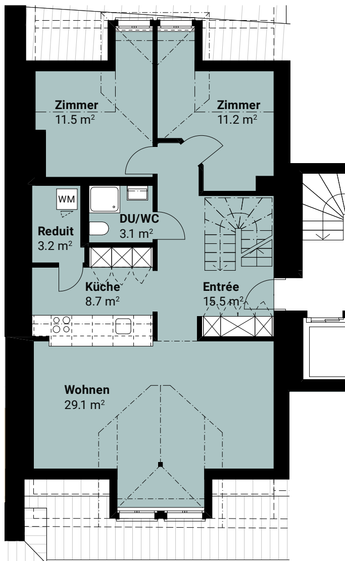
3. Obergeschoss
