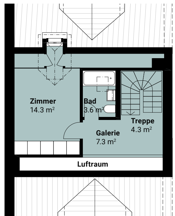
4. Obergeschoss
