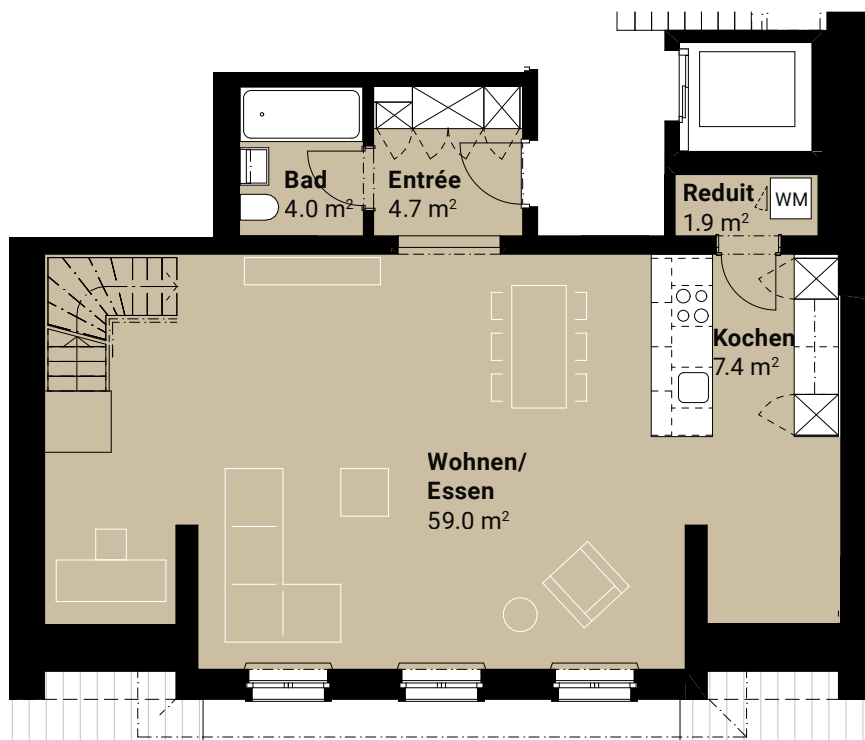
3. Obergeschoss
