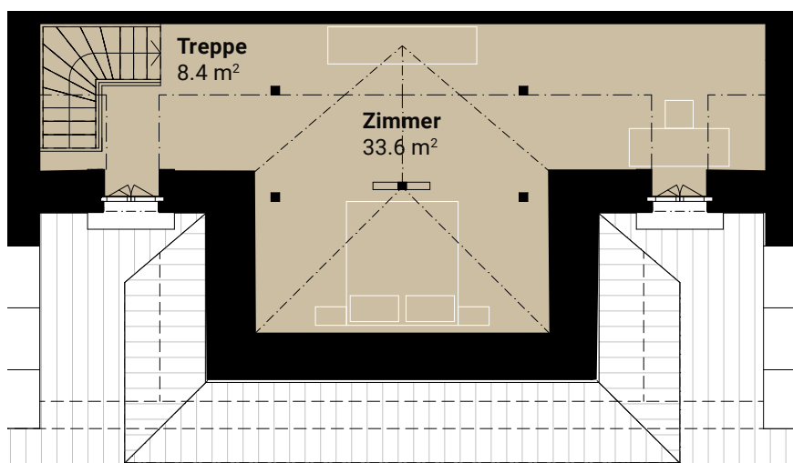
4. Obergeschoss
