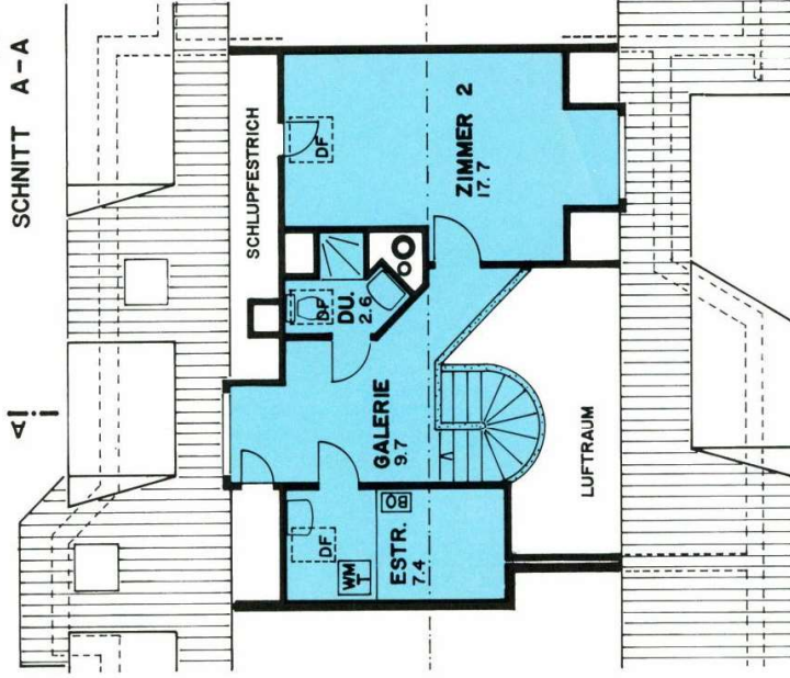
GRUNDRISS 2. DACHGESCHOSS
