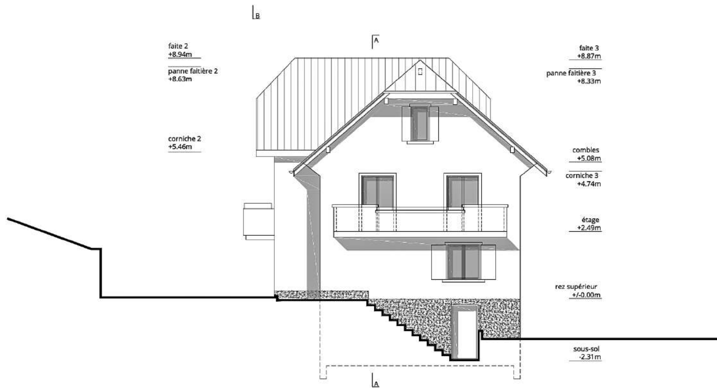
FAÇADE SUD OUEST
