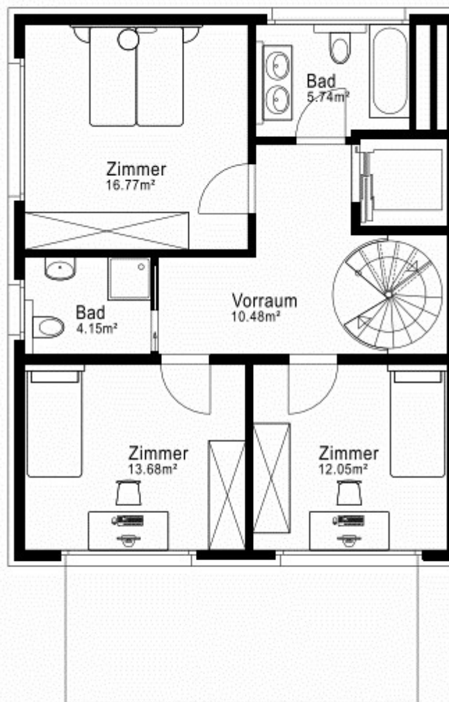
Obergeschoss
