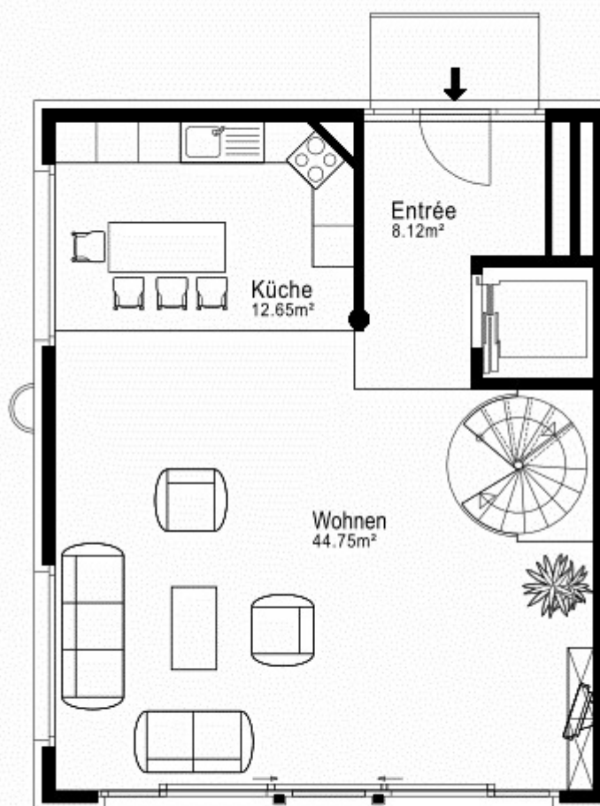
Erdgeschoss
