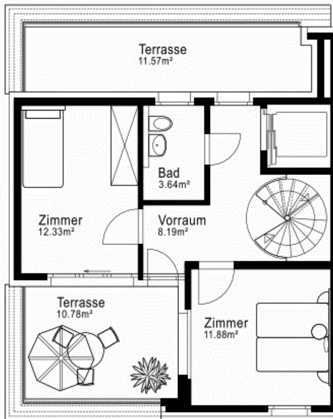
Dachgeschoss
