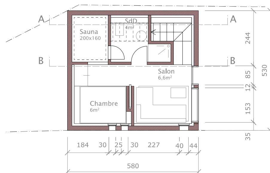
PLAN SOUS-SOL
