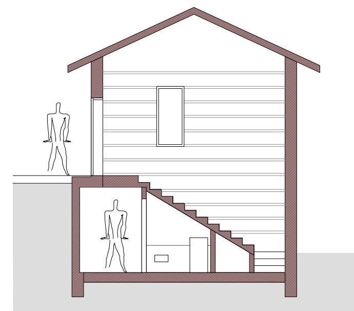
COUPE BB
