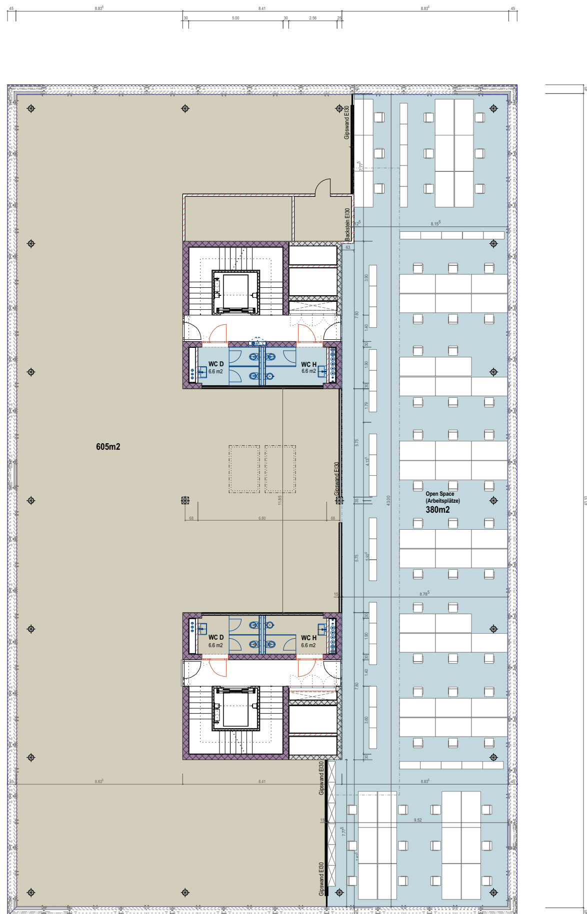
Grundriss / 1:200
