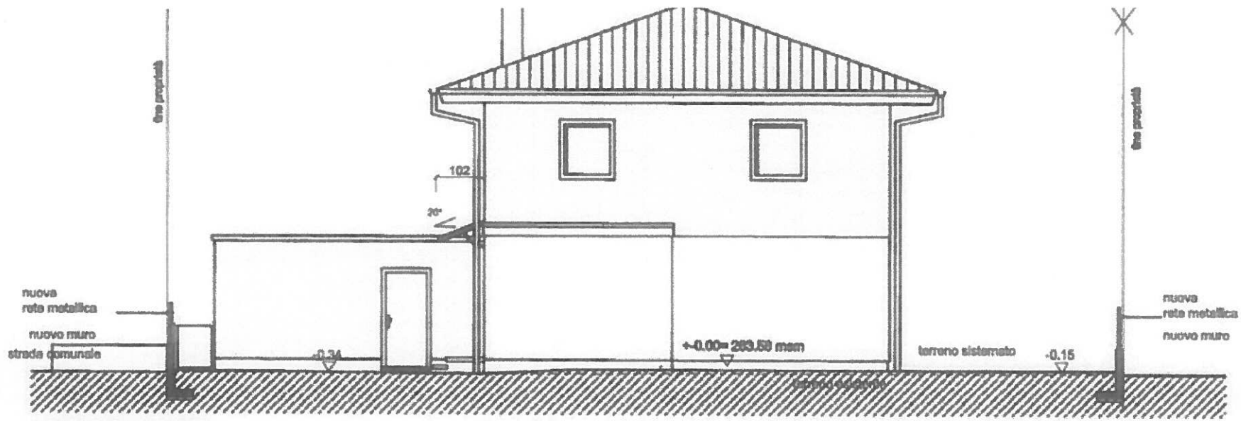
ANSICHT NORD
