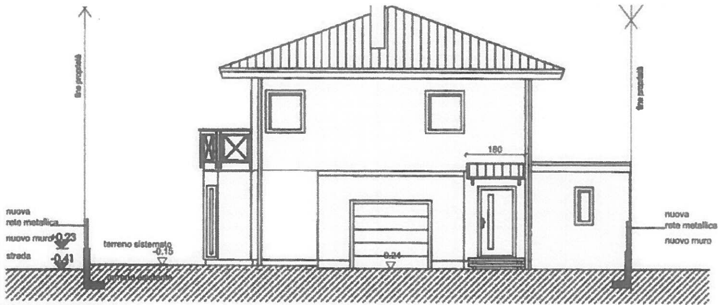
FACCIATA WEST
