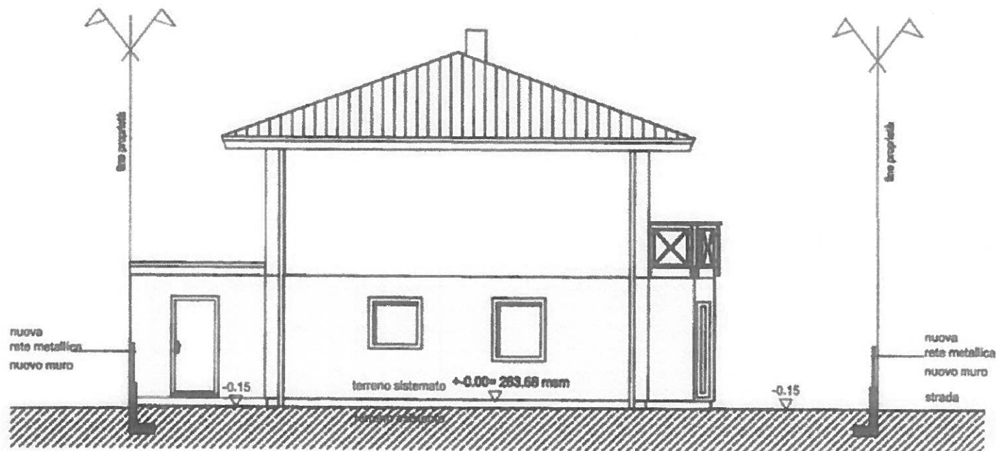
FACCIATA EST
