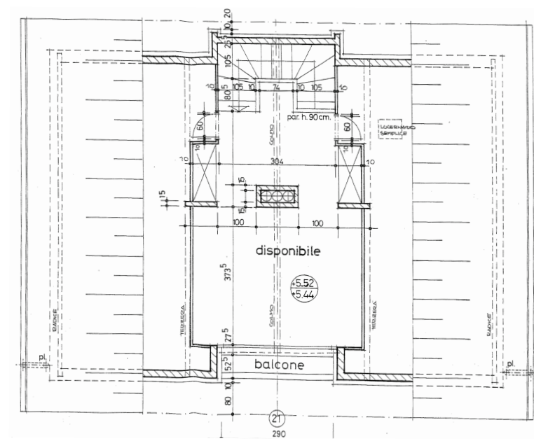
Pianta piano sottotetto
