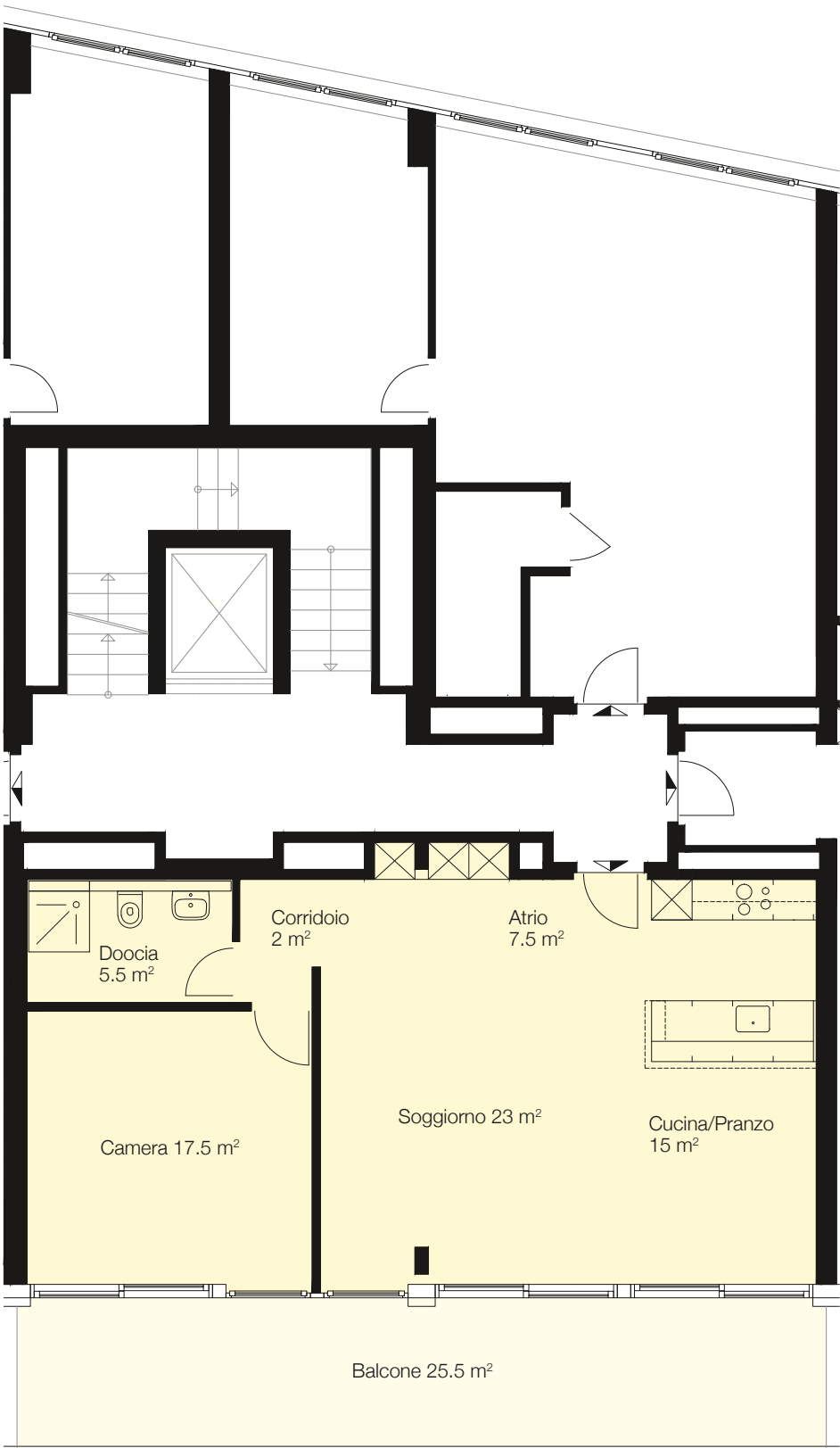
Pianta Scala 1:100
