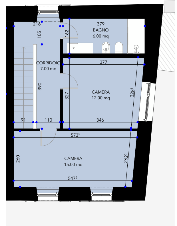
PIANO PRIMO Altezza locali da 3.20 a 4.30
