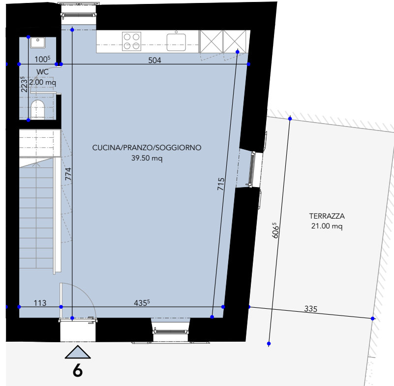
PIANO TERRA Altezza locali 3.19
