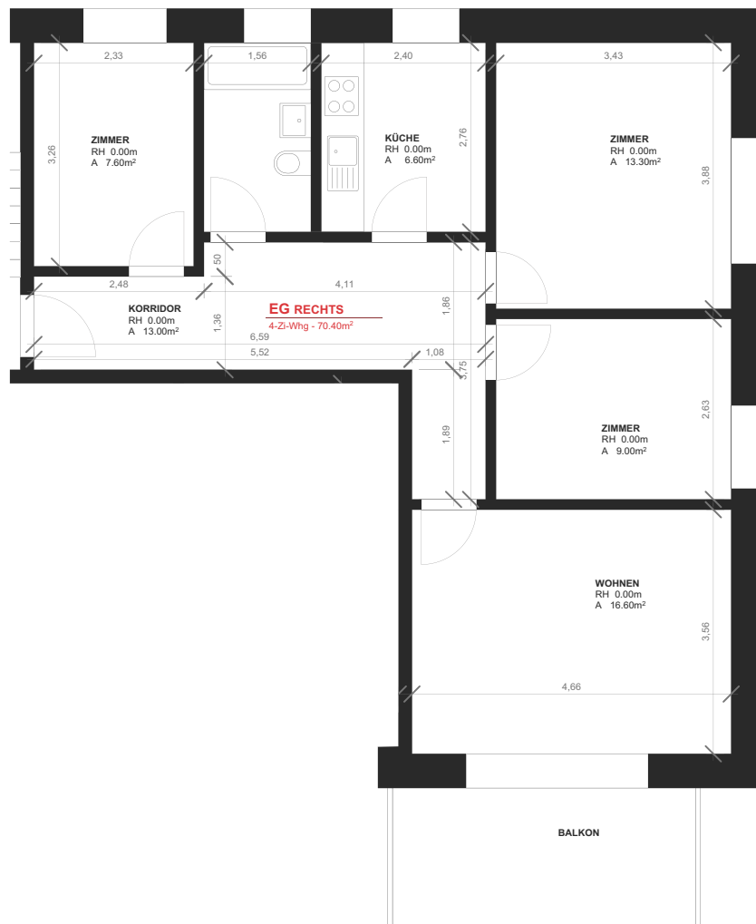
WOHNUNGSGRUNDRISS, 1:100
