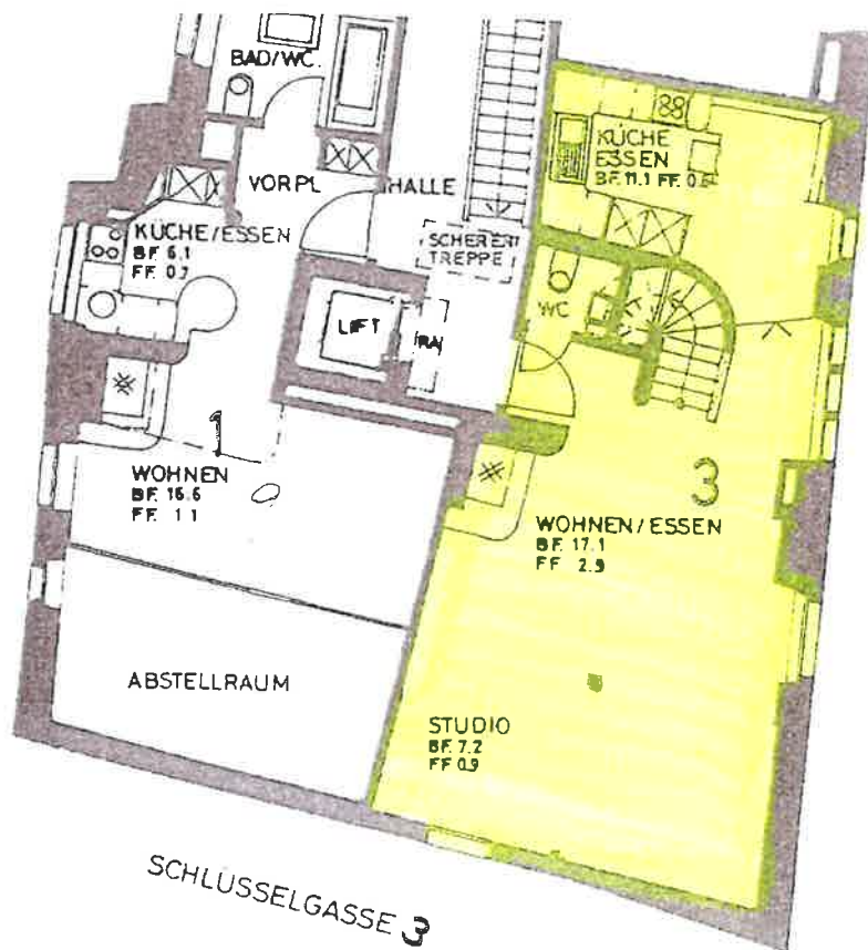
6. OBERGESCHOSS M.1:100
