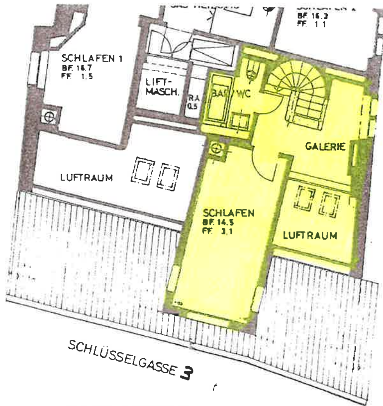
6. OBERGESCHOSS M.1:100
