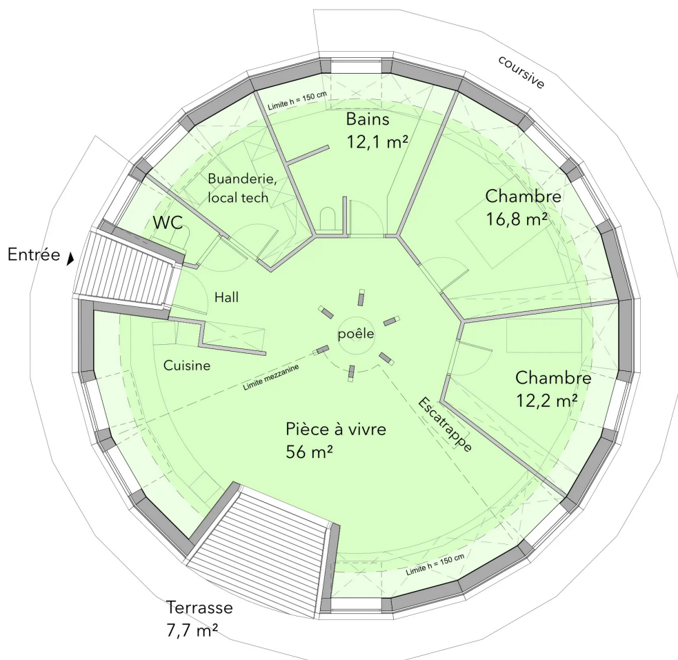
Rez-de-chaussée
