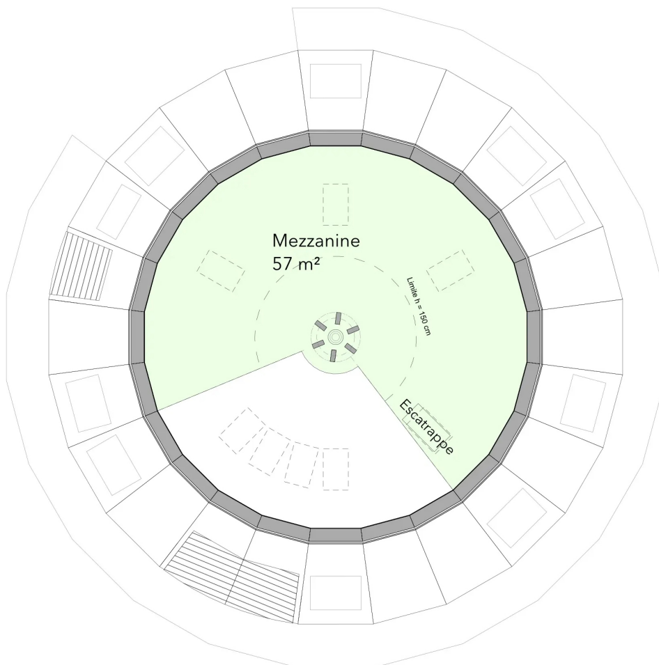
Étage
