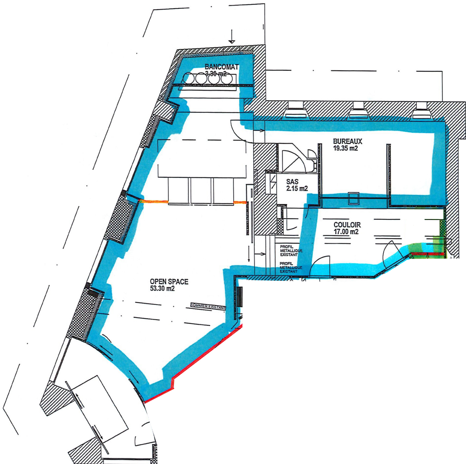
PLAN DU REZ-DE-CHAUSSEE
