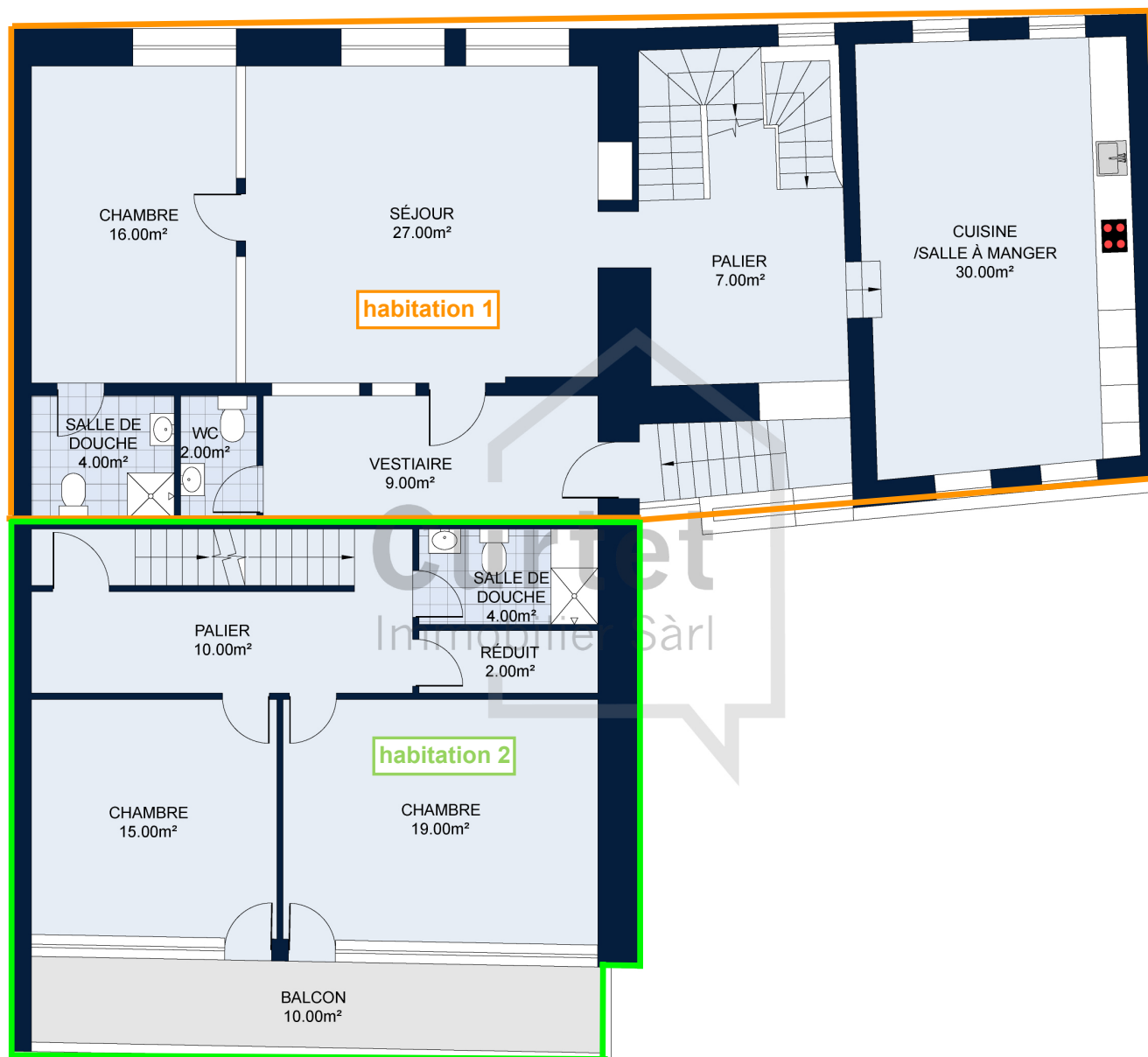
PREMIER ÉTAGE
