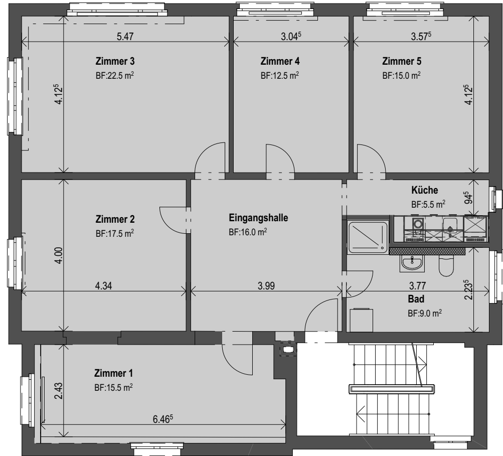
1. OBERGESCHOSS, Mst. 1:100
