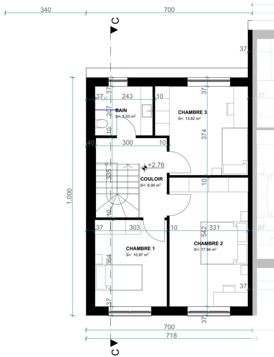
ETAGE 1 1/100 S=: 70.00 m²
