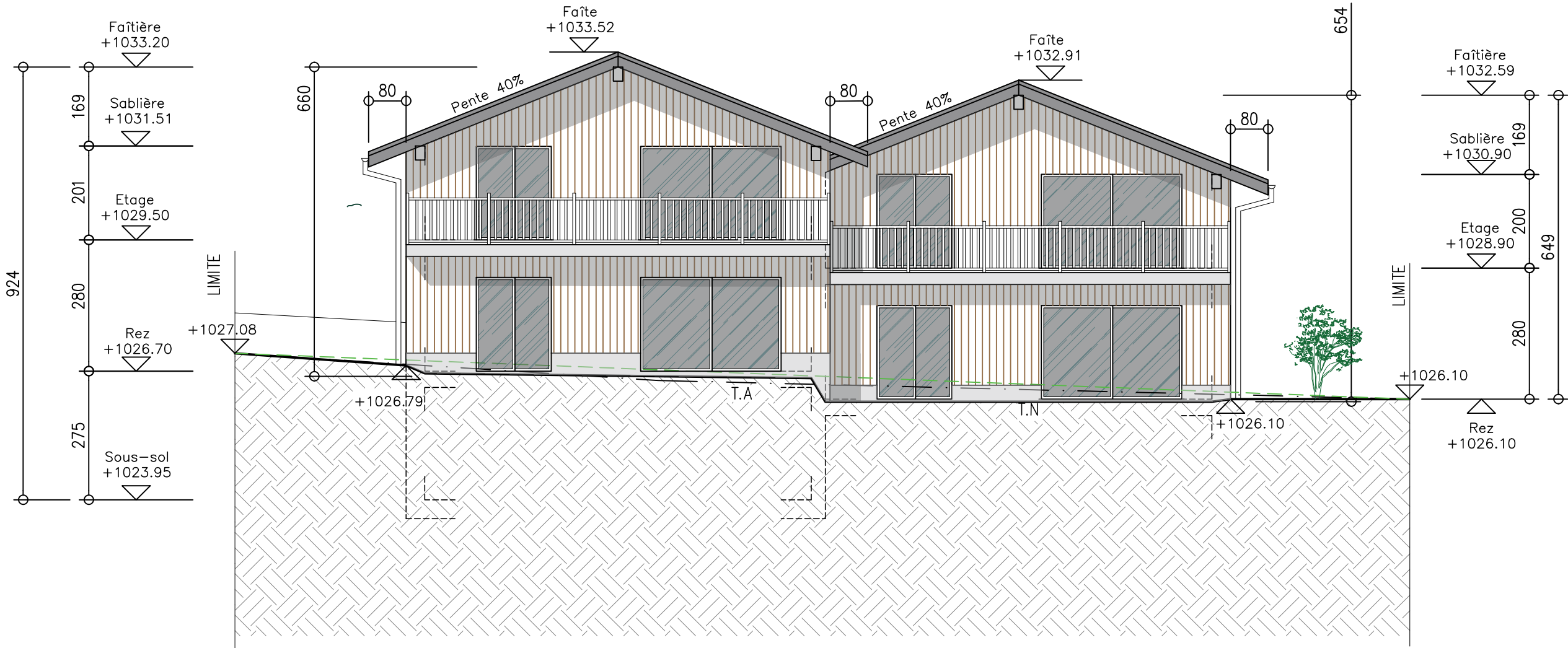
Façade Nord – Bâtiment A
