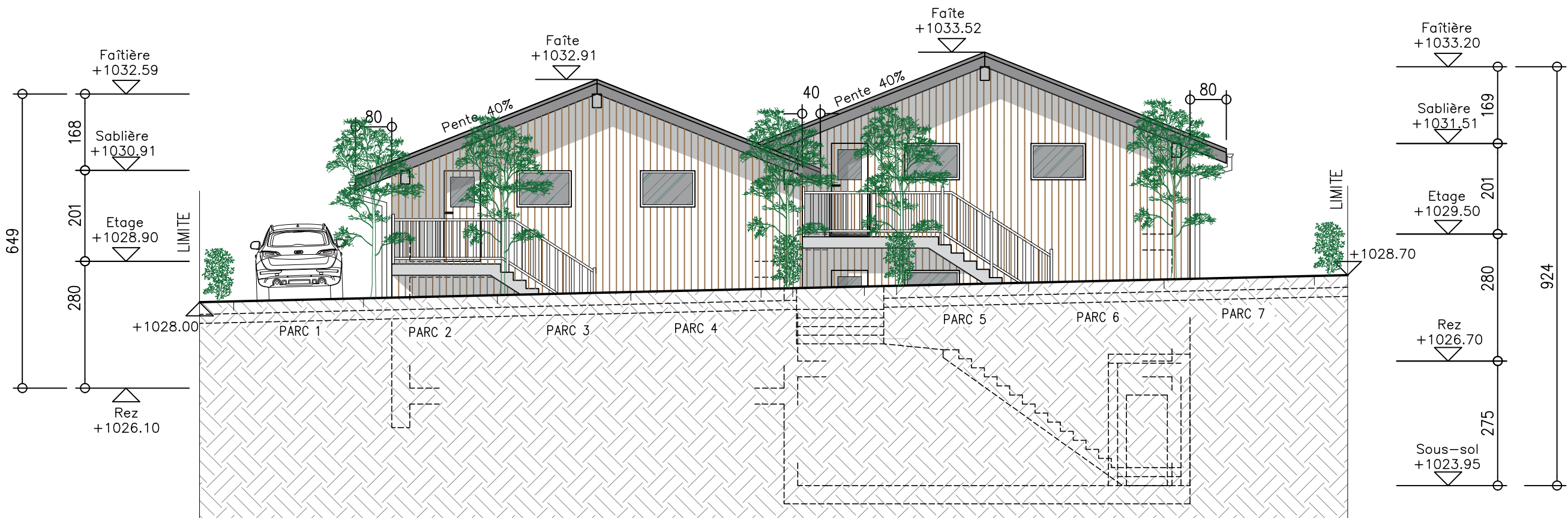
Façade Sud – Bâtiment A
