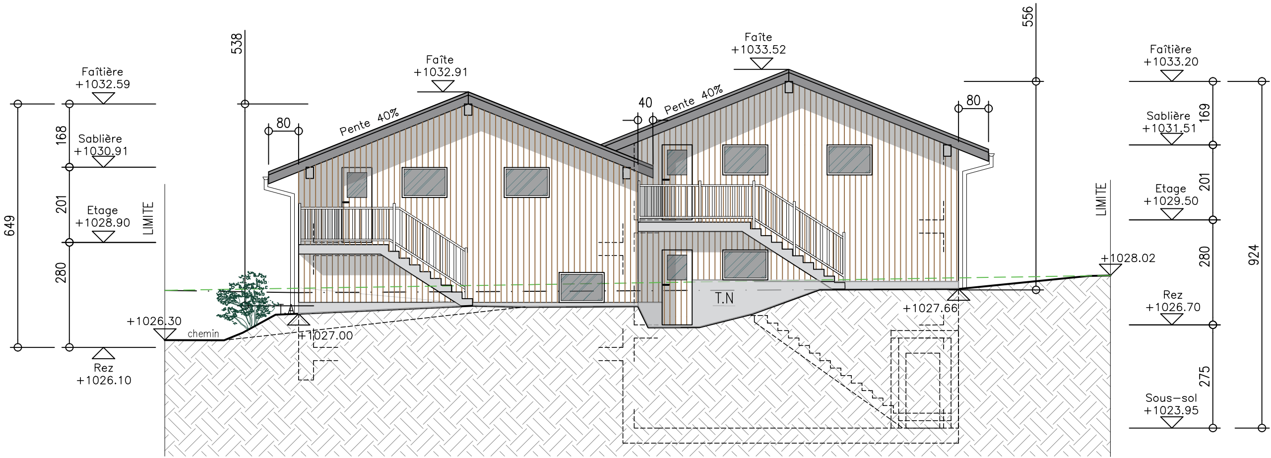
Façade Sud – Bâtiment A
