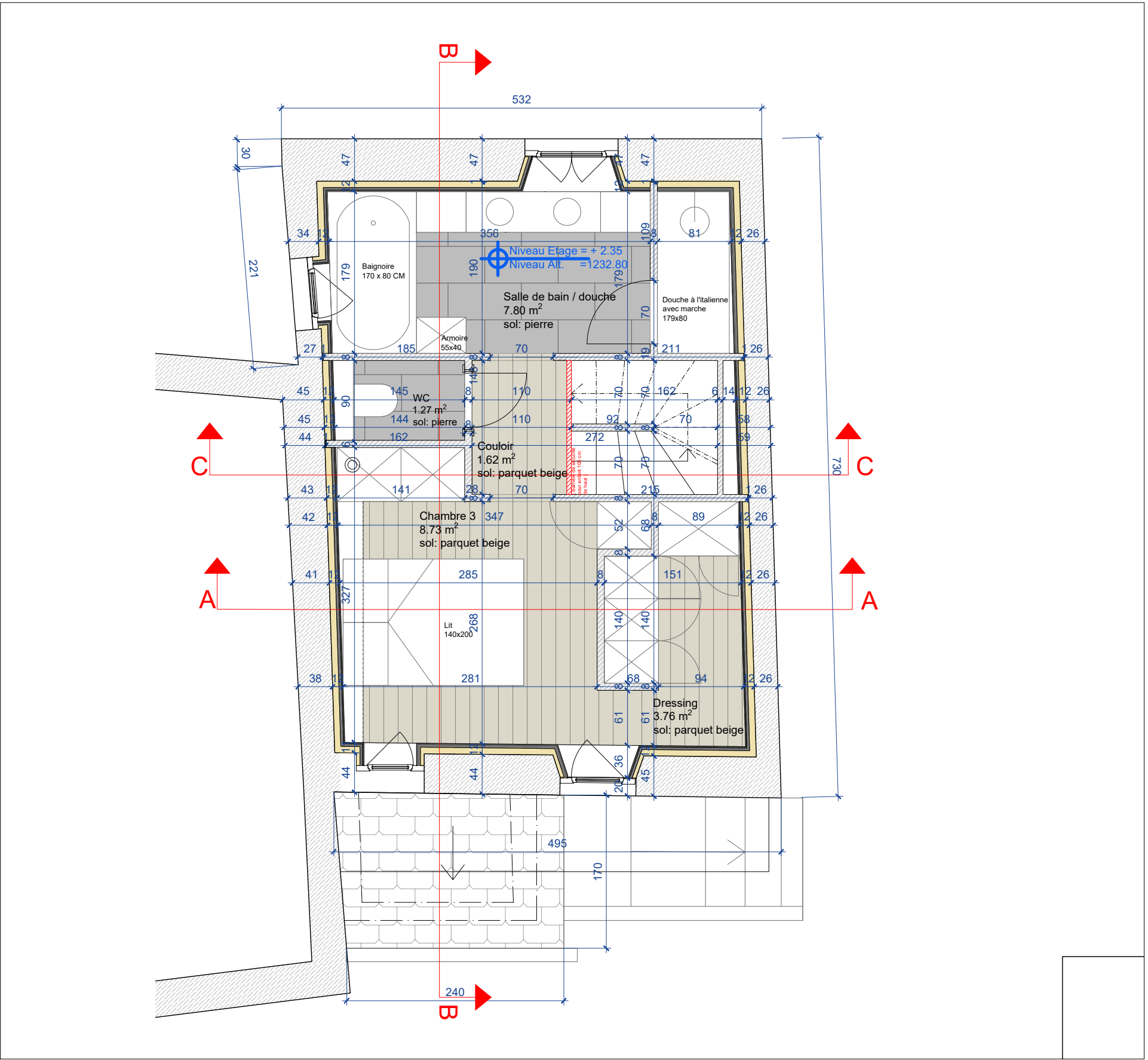
Plan Etage
