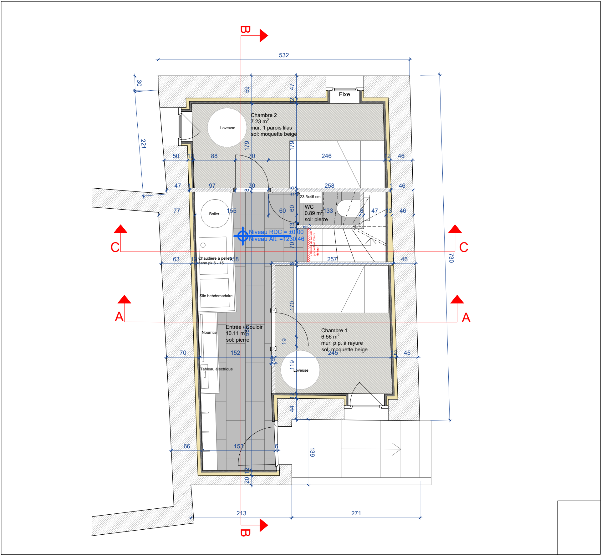
Plan RDC
