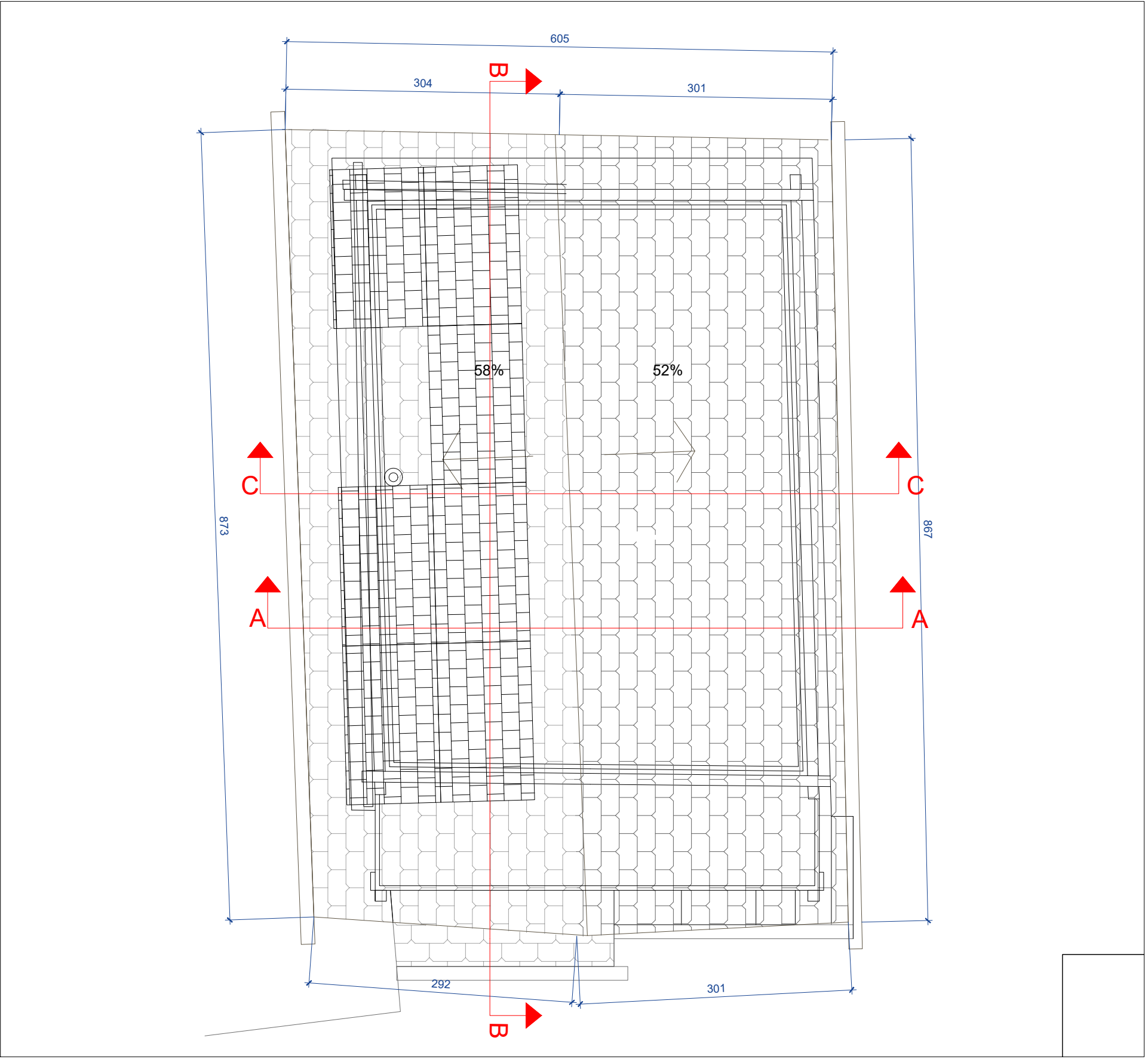
Plan Toiture
