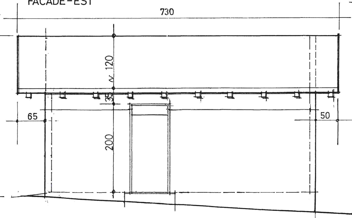
FACADE-EST
