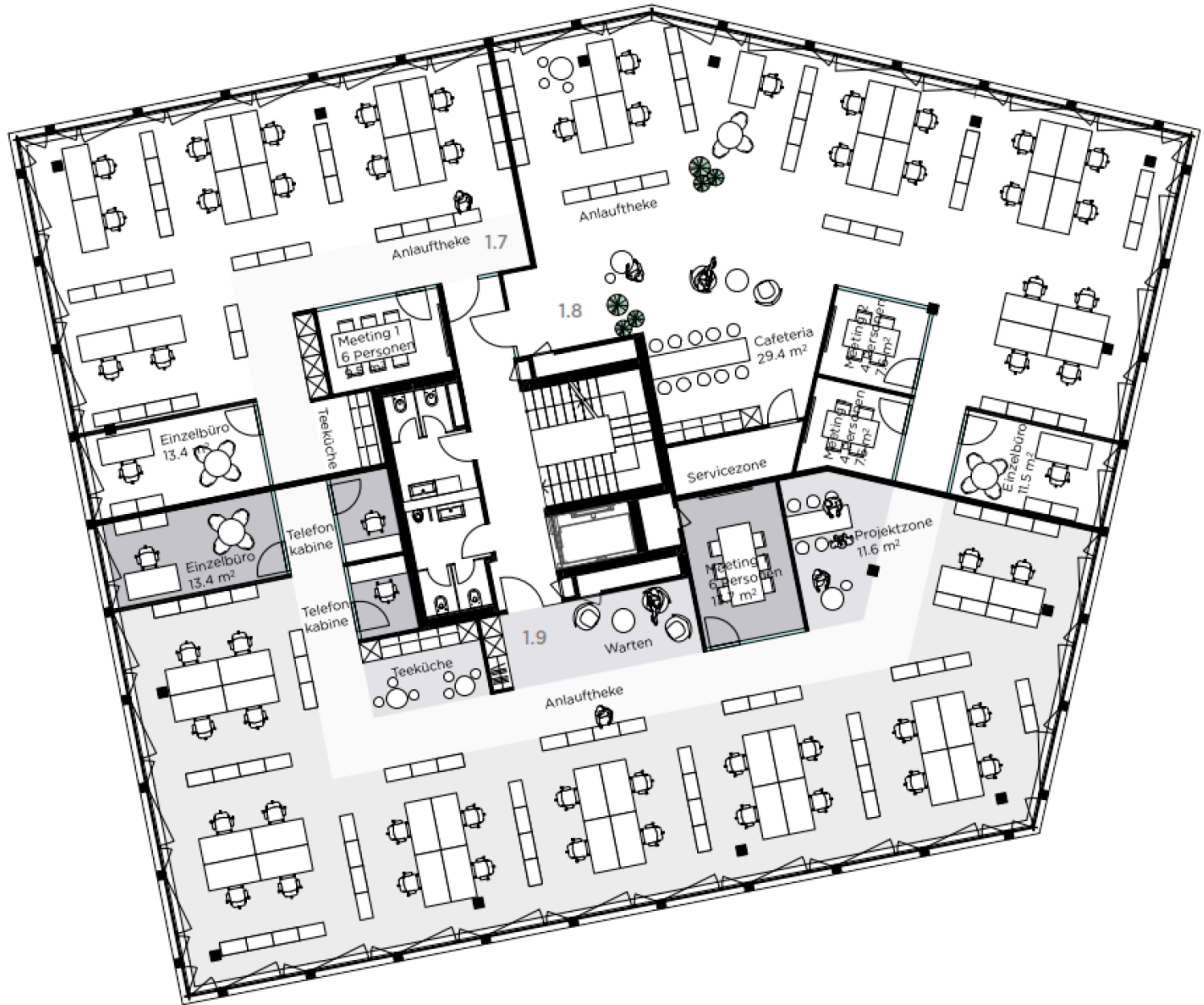
Layoutvorschlag 2. OG
