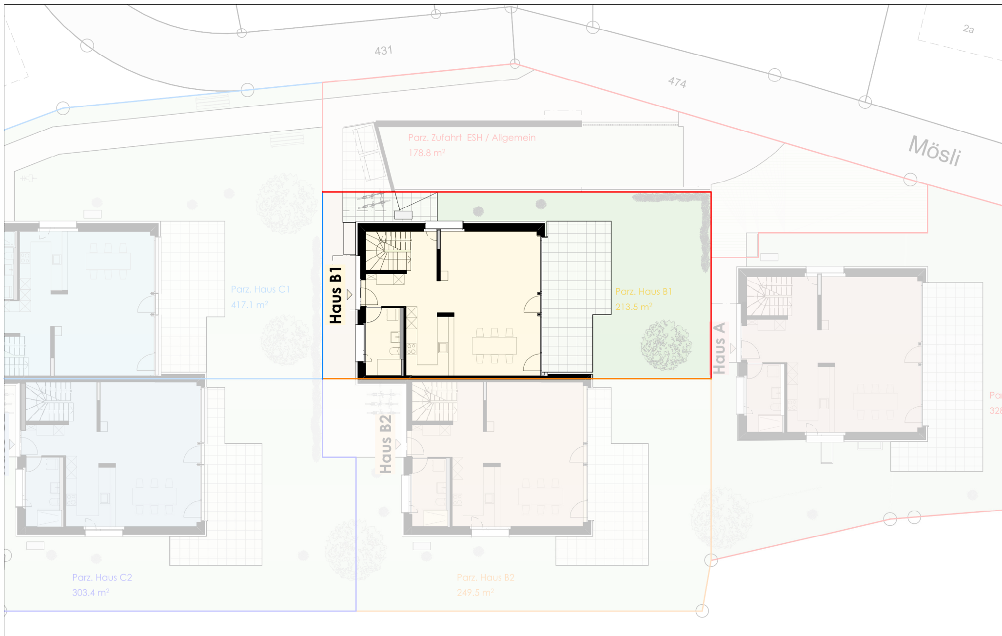
Haus B1 Grundriss EG mit Umgebung
