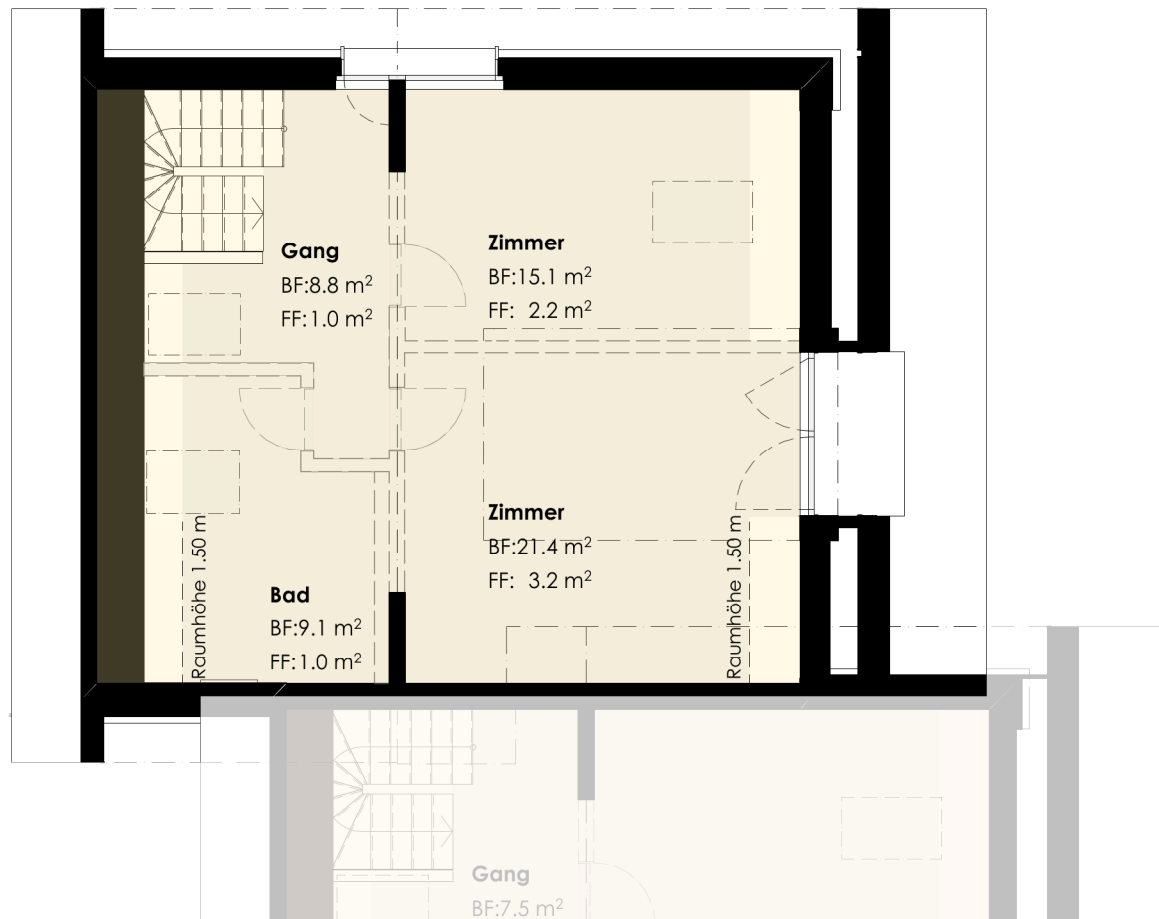
Haus B1 Grundriss Dachgeschoss (nicht ausgebaut)
