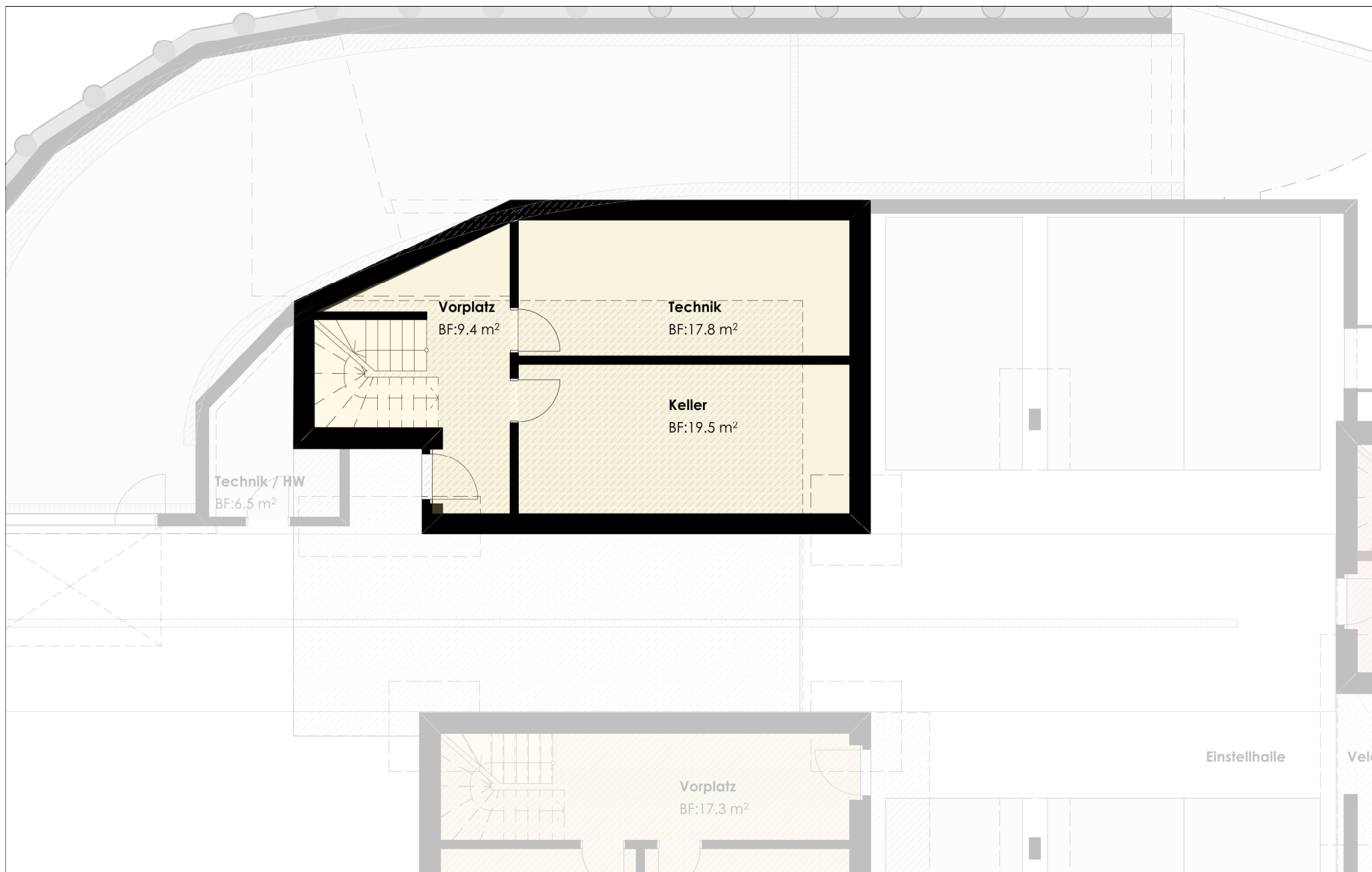
Haus B1 Grundriss Untergeschoss
