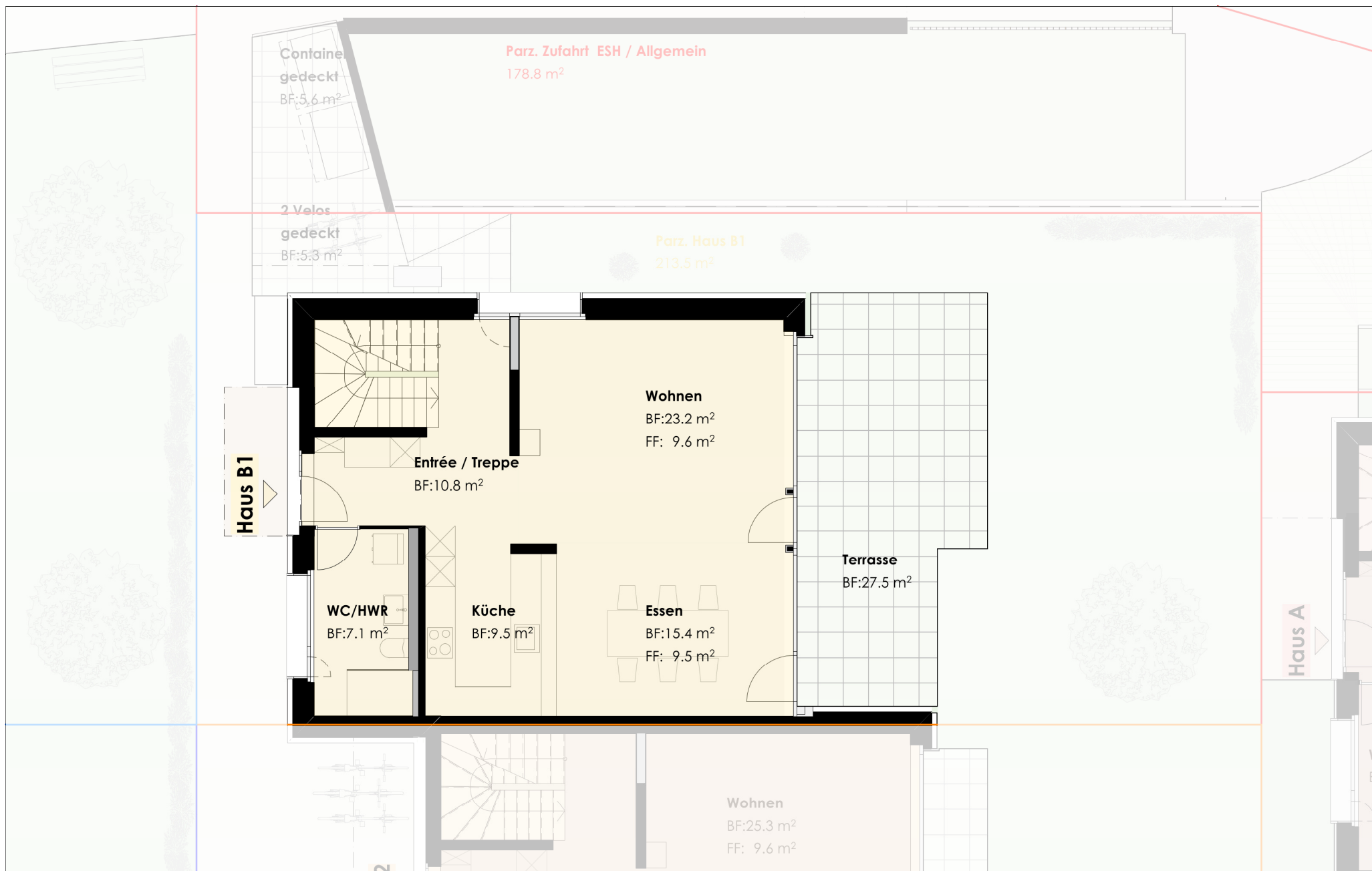
Haus B1 Grundriss Erdgeschoss
