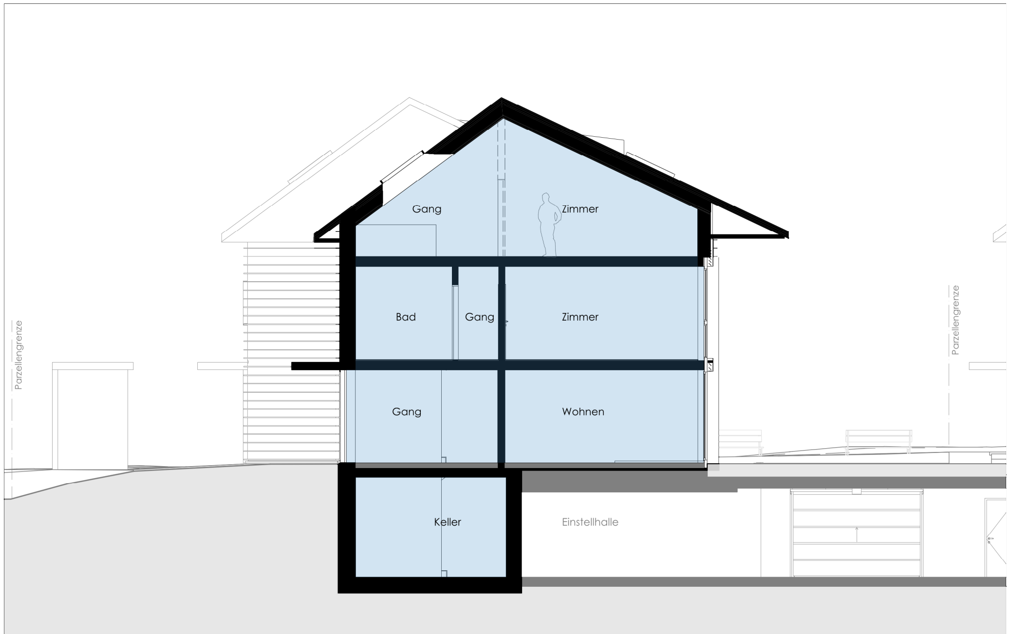
Haus C2 Querschnitt
