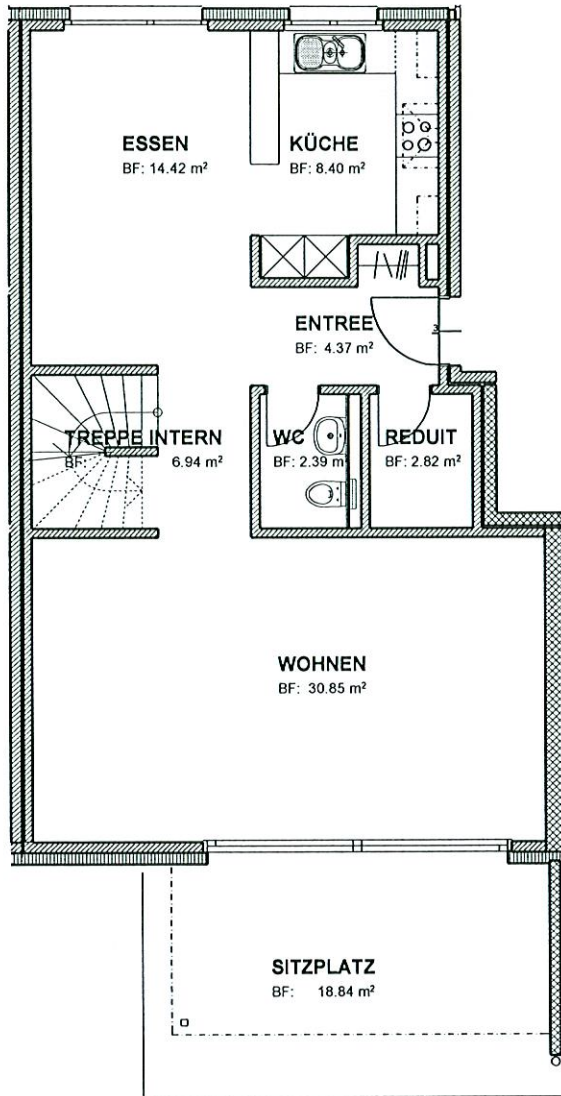
ERDGESCHOSS
