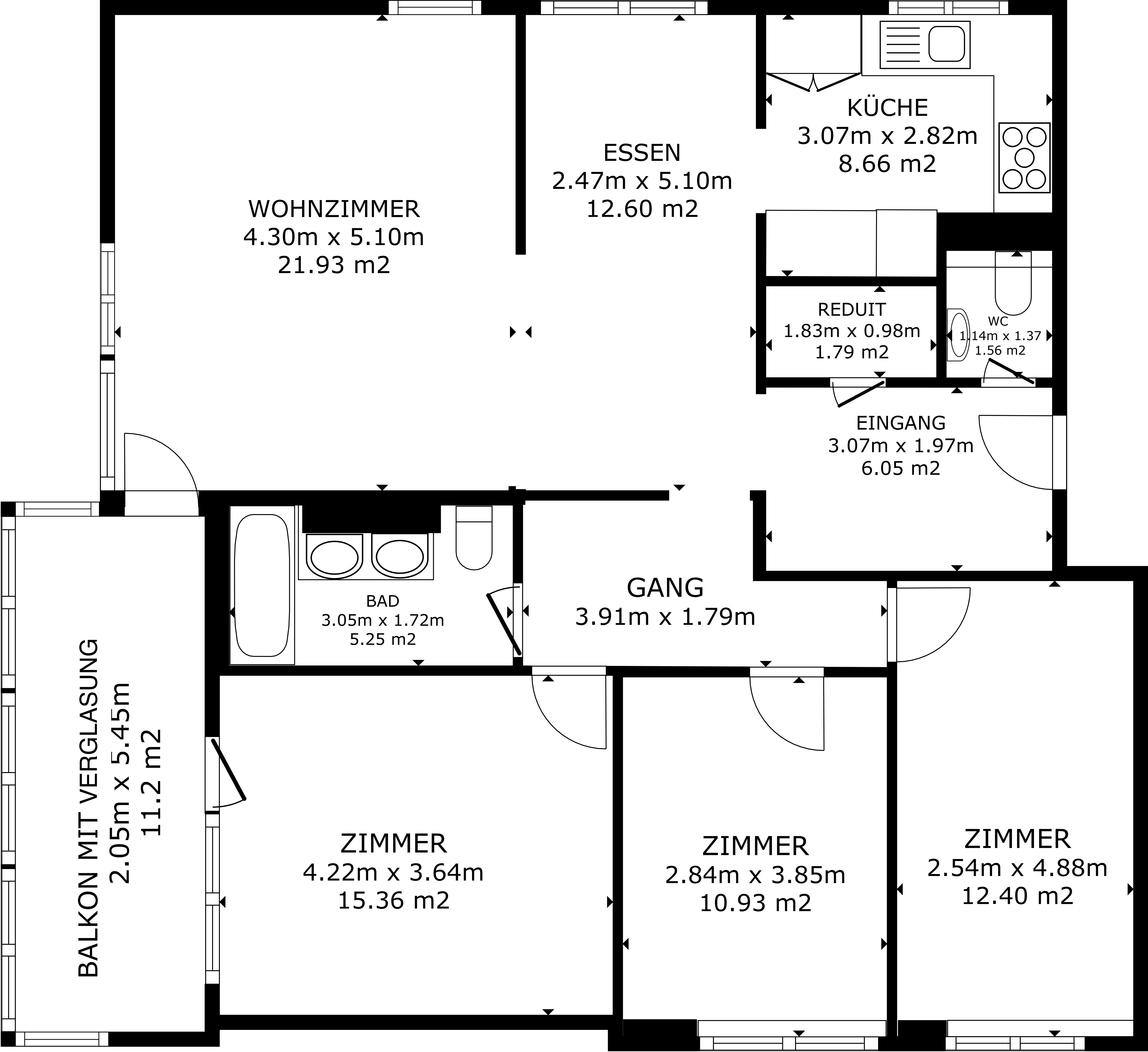
GRUNDRISS
