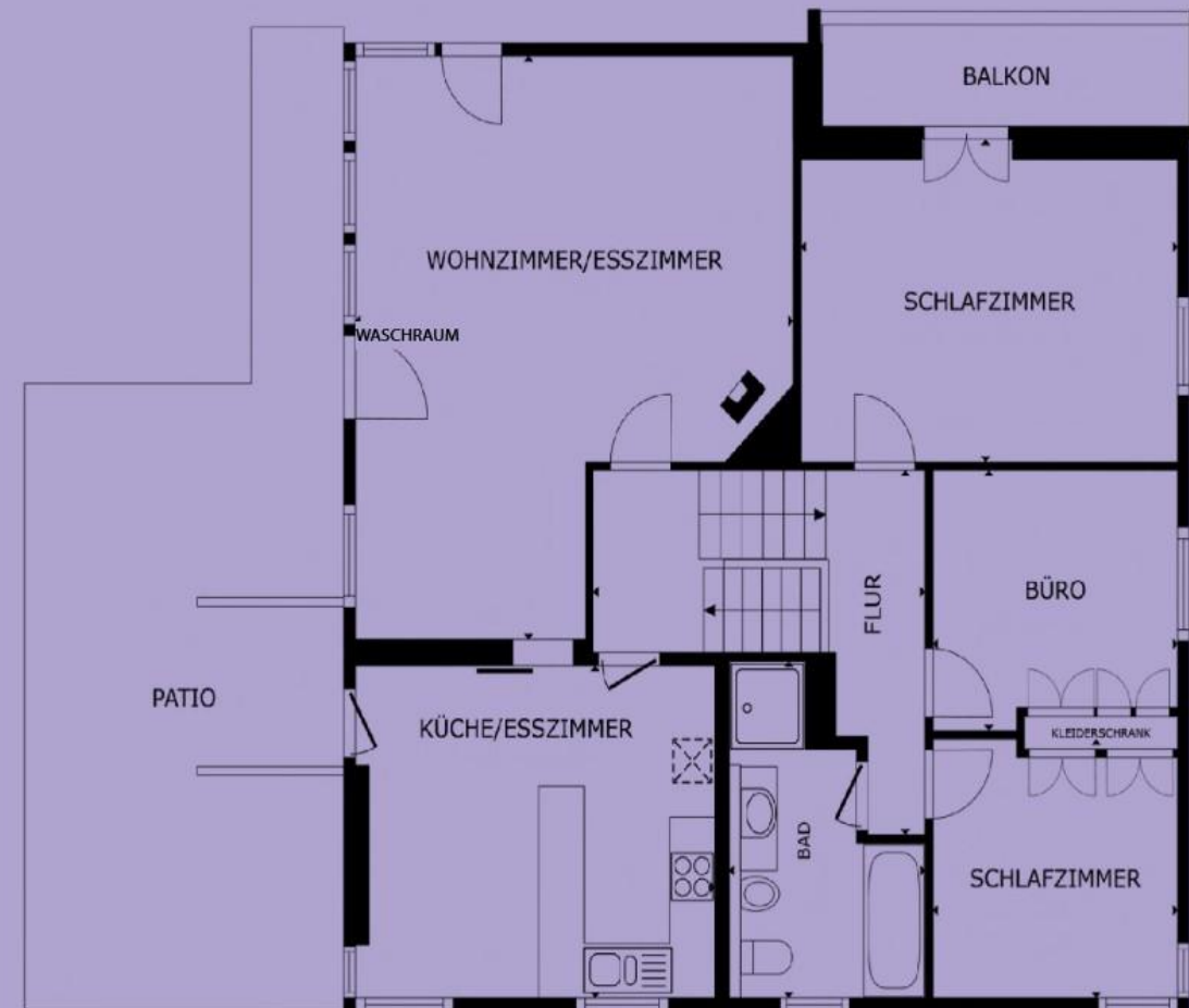
Erdgeschoss/Obergeschoss
