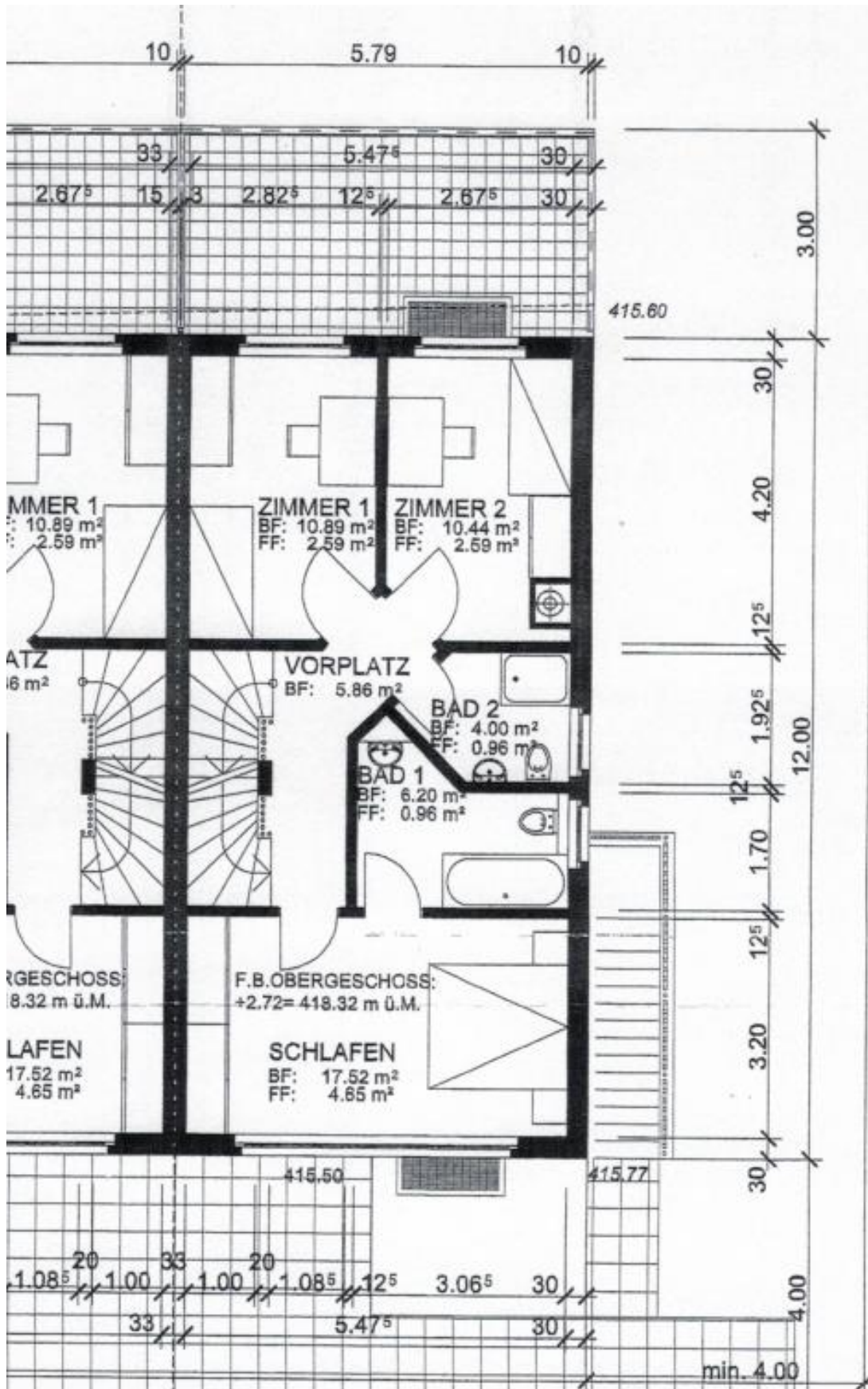
1. Obergeschoss
