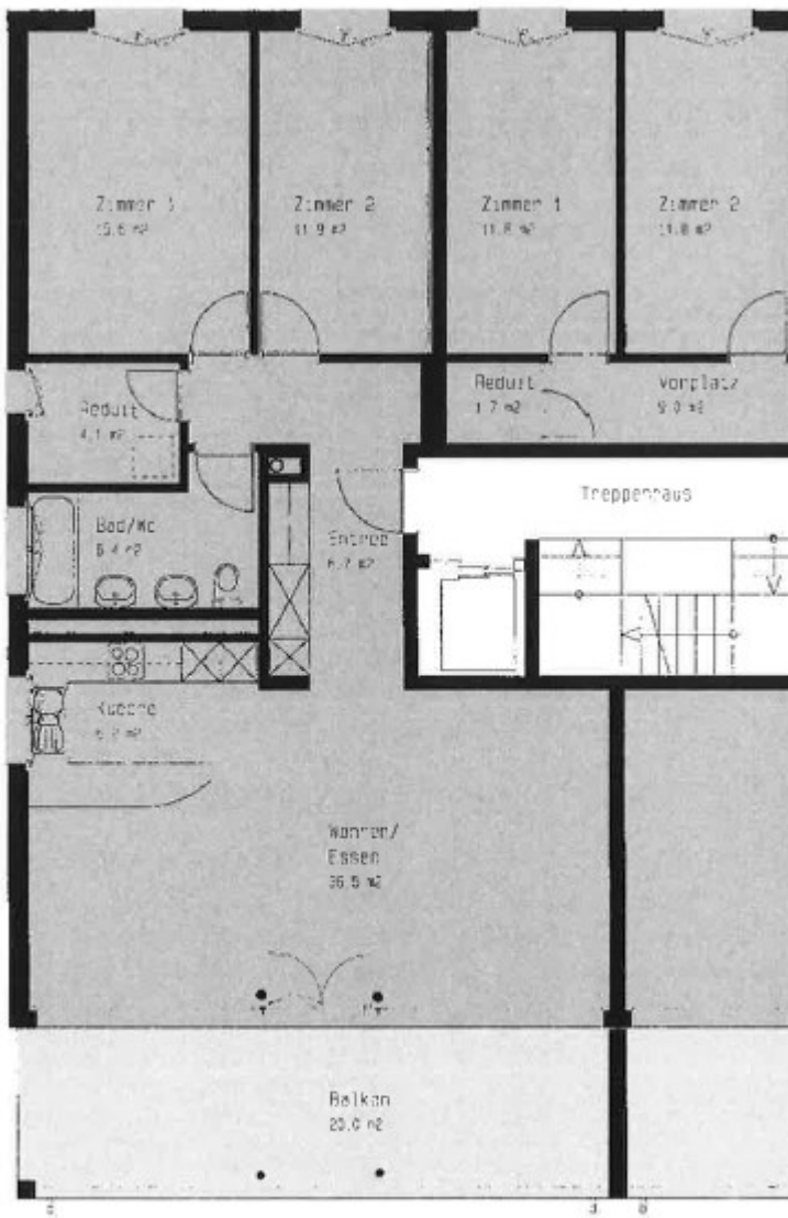
3 1/2-Zimmer-Wohnung
