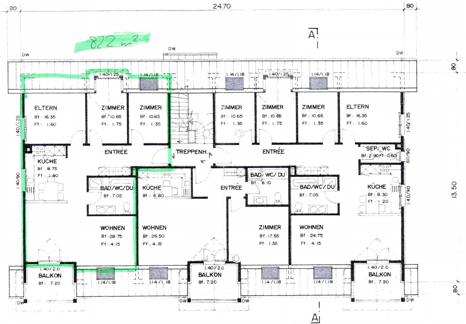
GRUNDRISS DACHGESCHOSS
