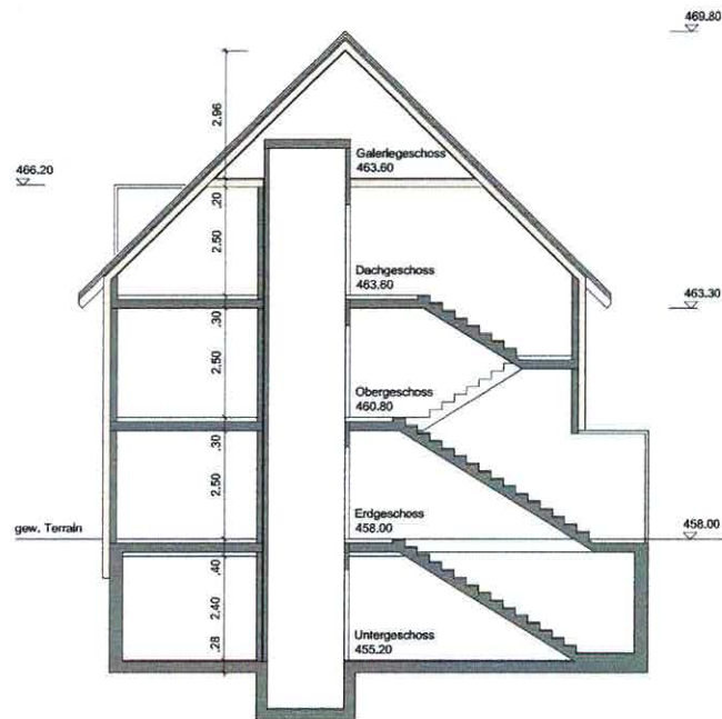
Schnitt A-A Gebäude B
