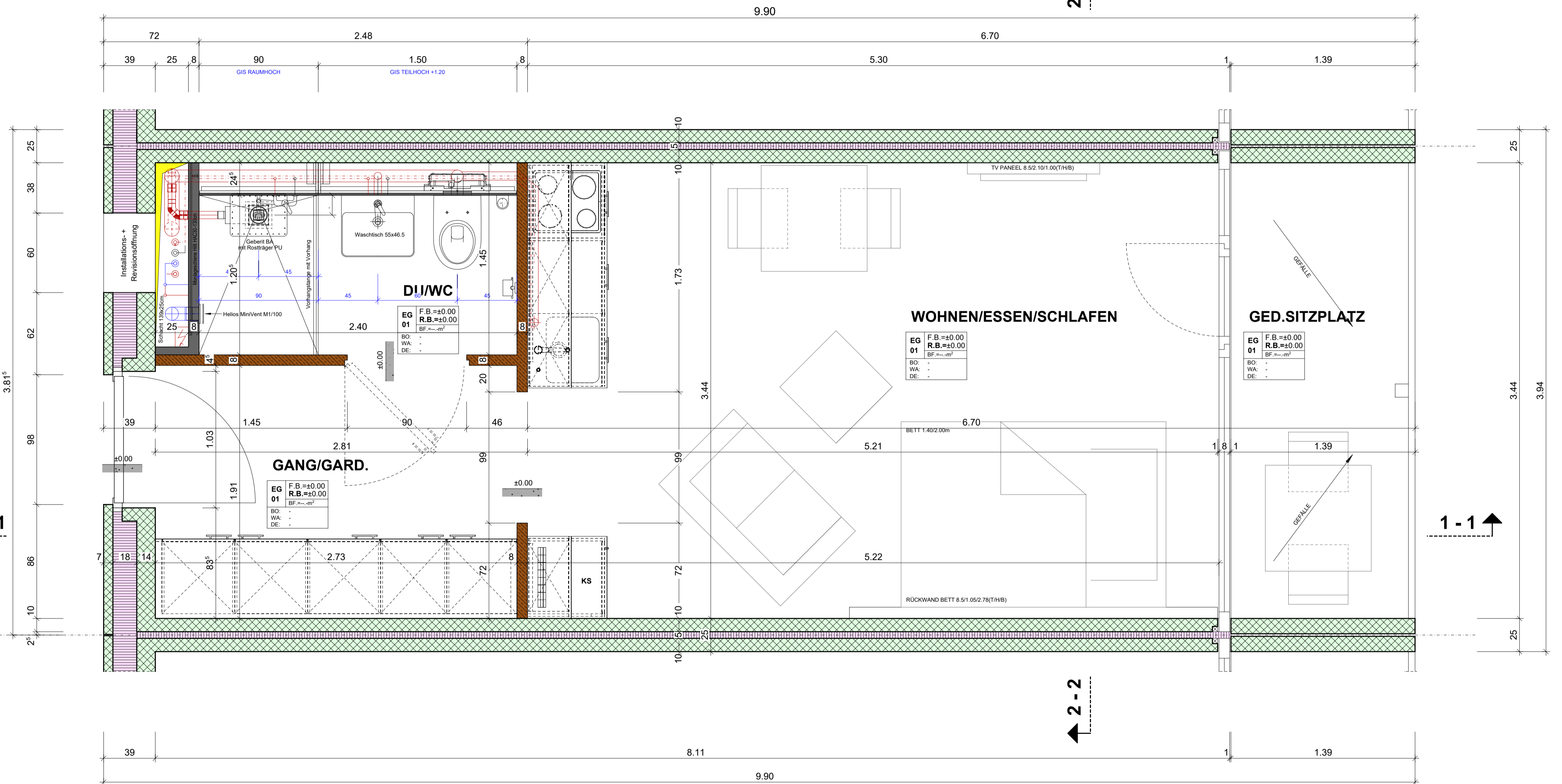
G R U N D R I S S 1:20 (ZWISCHENELEMENT)
