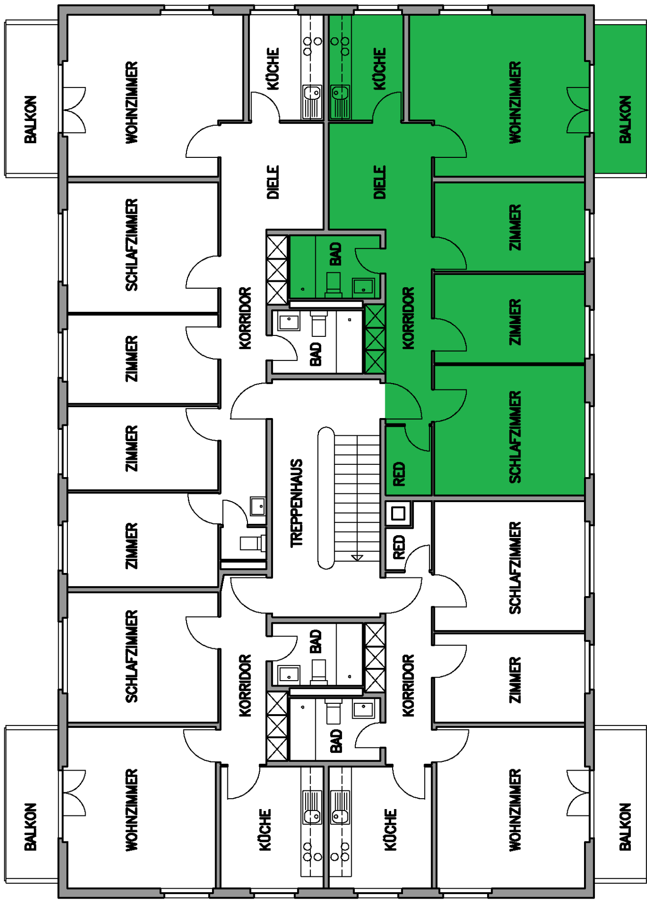
1. OBERGESCHOSS 1:100 HAGMANNSTRASSE 1, 4565 RECHERSWIL
