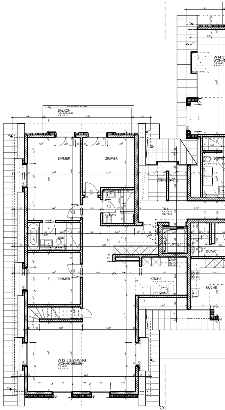
DACHGESCHOSS
