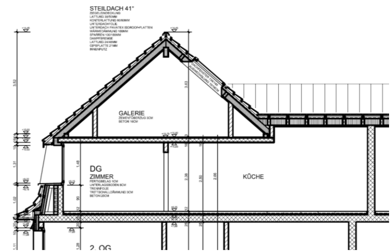
SCHNITT
